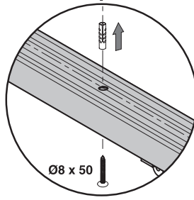
[A] Rechtstreeks tegen het plafond: de motor wordt rechtstreeks met de rail tegen het plafond gemonteerd
